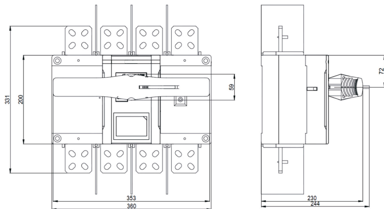
ГАБАРИТНЫЕ РАЗМЕРЫ ВН-IS-AKSOL 1250 AF СО СТАЦИОНАРНОЙ РУКОЯТКОЙ
