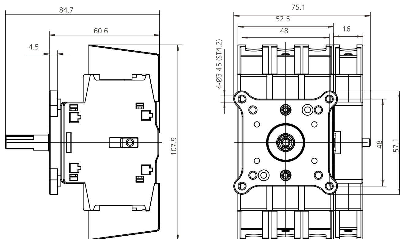
80AF-4P с KBB
