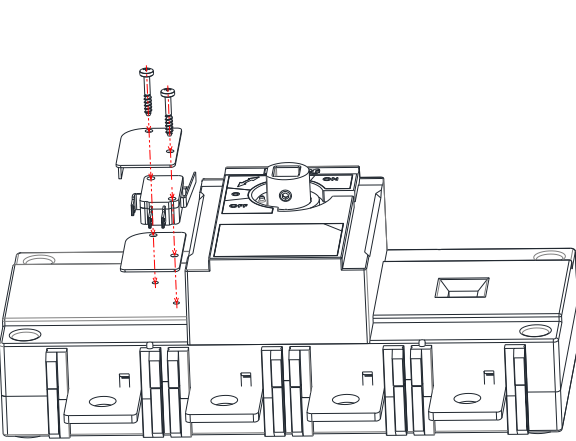
Установка 1 доп. контакта
