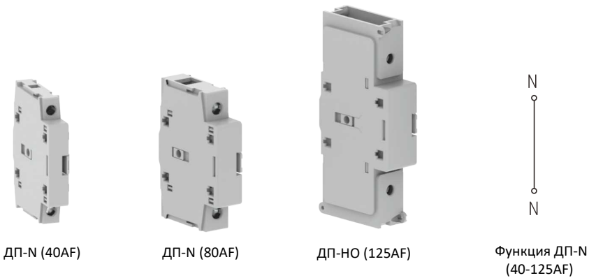
Дополнительные полюсы N 40-125AF
