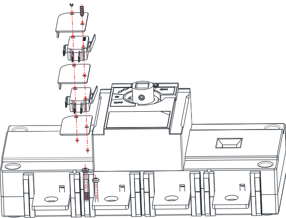
Установка 2 доп. контактов
