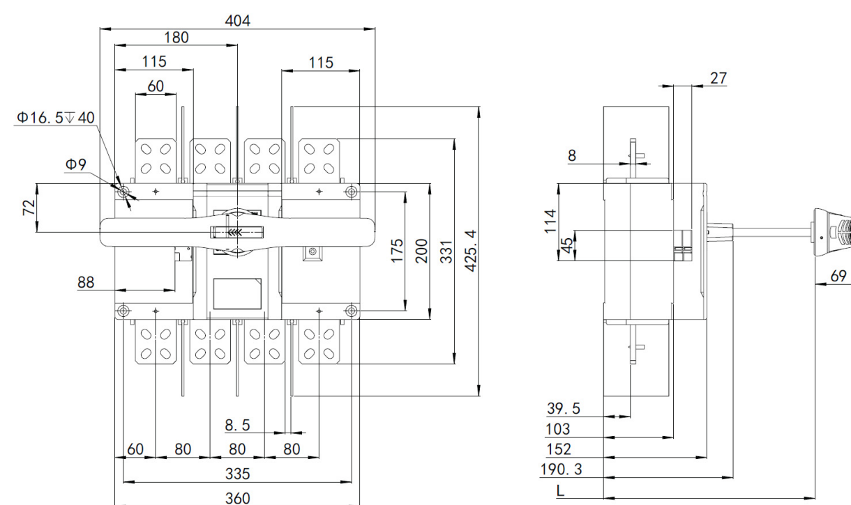
ГАБАРИТНЫЕ РАЗМЕРЫ ВН-IS-AKSOL 1250 AF С ВЫНОСНОЙ РУКОЯТКОЙ
