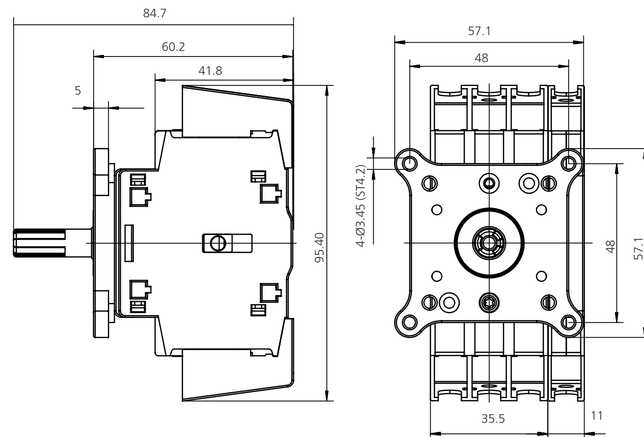
40AF-4P с KBB
