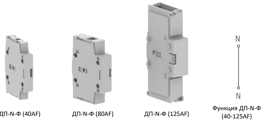
Дополнительные полюсы N для выключателей фронтального монтажа 40-125AF
