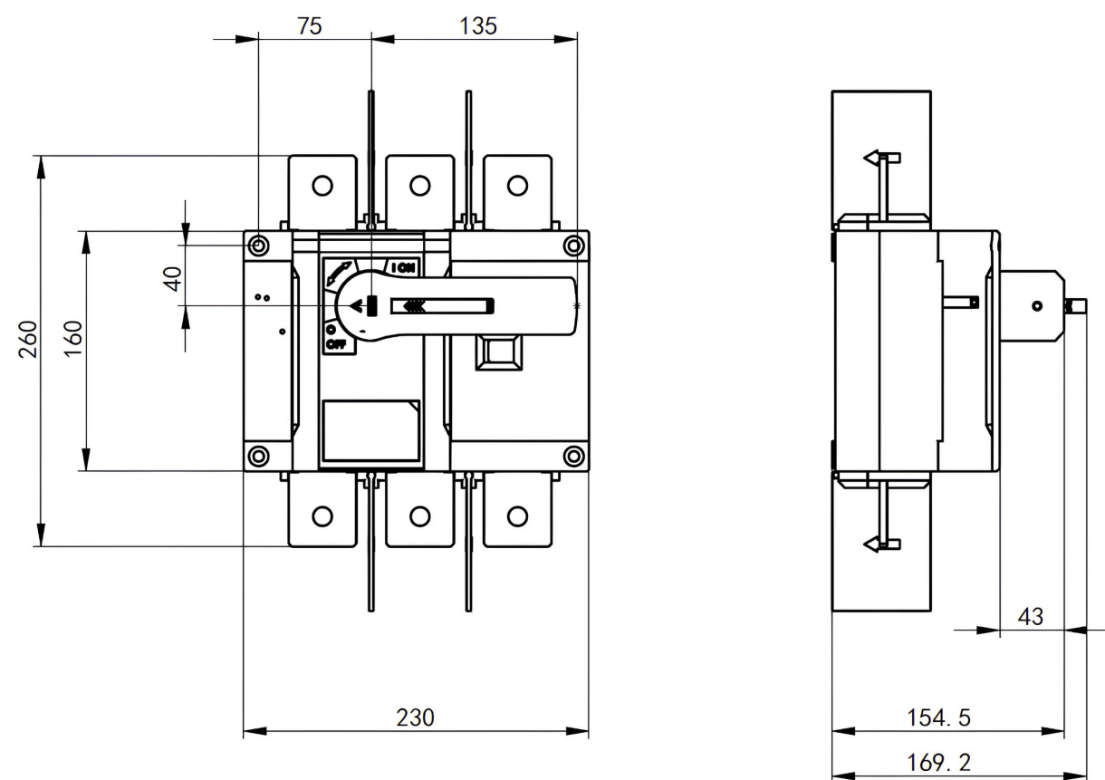
ГАБАРИТНЫЕ РАЗМЕРЫ ВН-IS-AKSOL 1250 AF СО СТАЦИОНАРНОЙ РУКОЯТКОЙ
