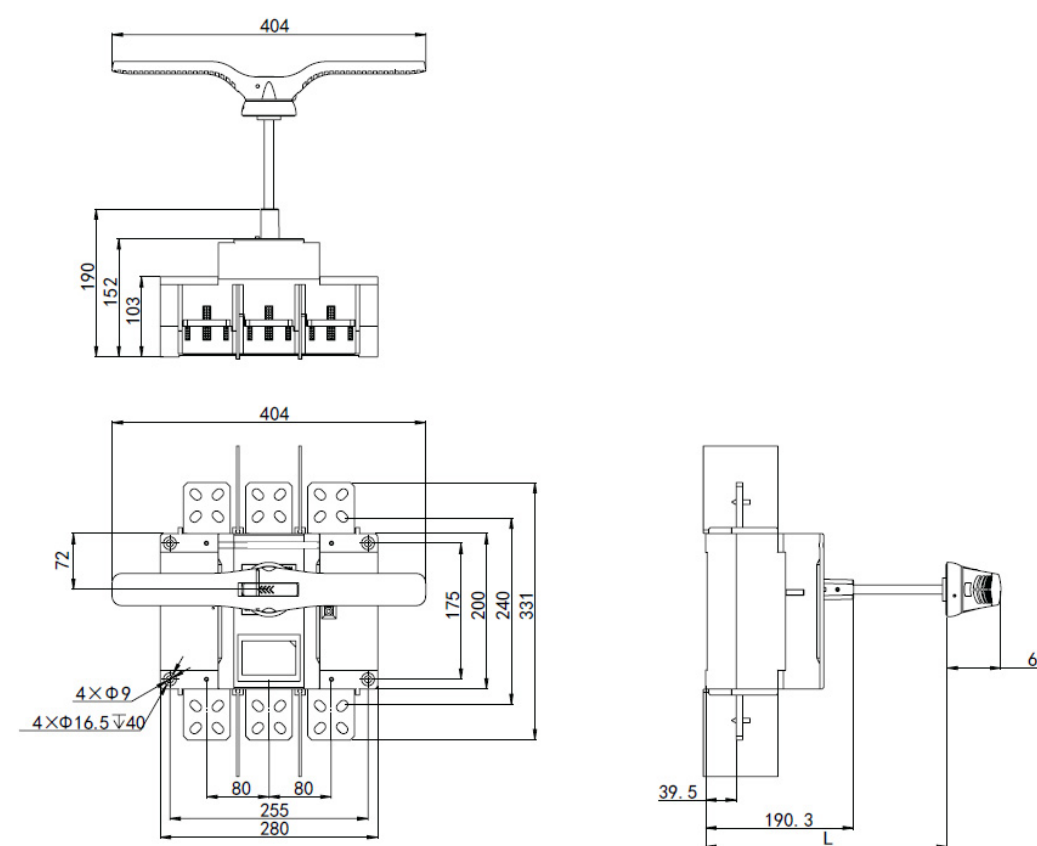
ГАБАРИТНЫЕ РАЗМЕРЫ ВН-IS-AKSOL 1250 AF С ВЫНОСНОЙ РУКОЯТКОЙ
