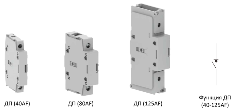
Дополнительные полюсы 1P 40-125AF
