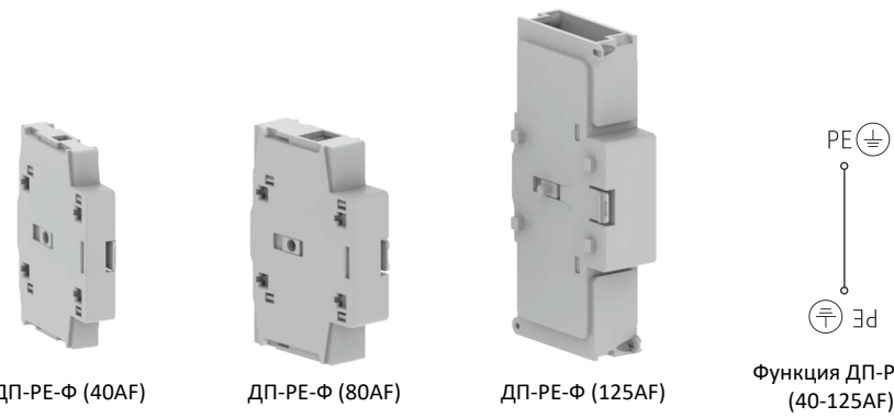
Дополнительные полюсы PE для выключателей фронтального монтажа 40-125AF
