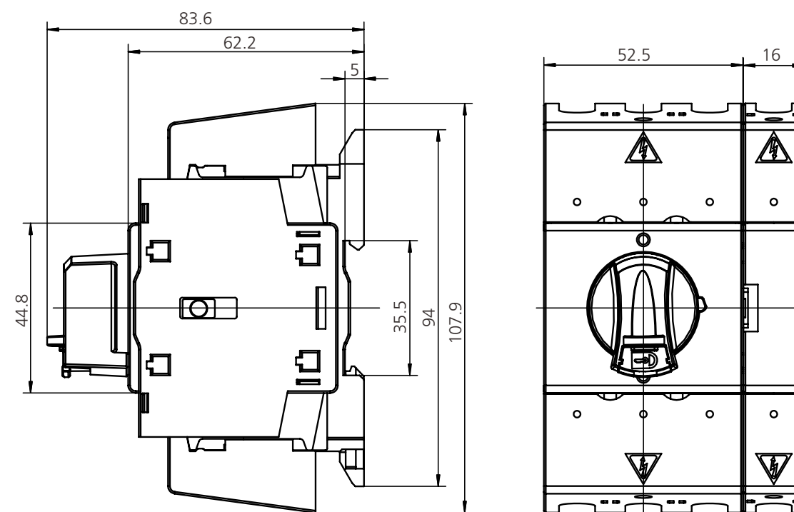
80AF-4P с KBB
