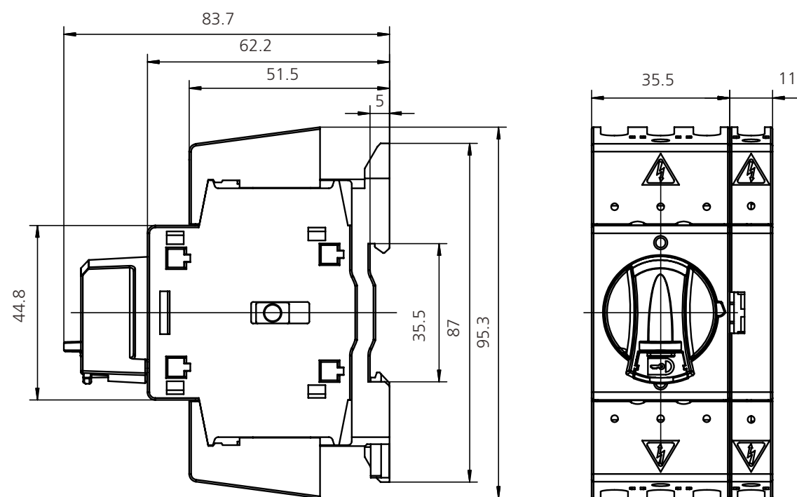
40AF-4P с KBB (изолирующие крышки выводов)
