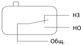
Электрическая схема доп. контакта (250-2000AF)
