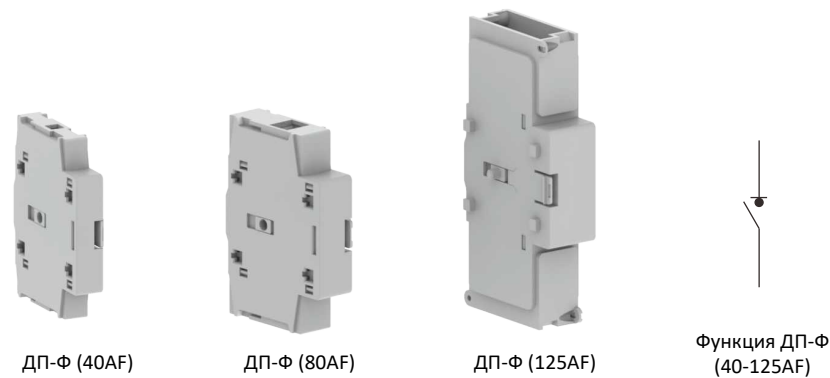
Дополнительные полюсы 1P для выключателей фронтального монтажа 40-125AF
