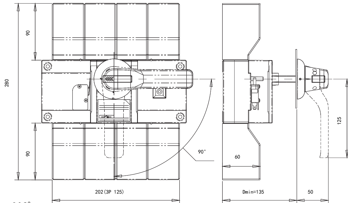
ГАБАРИТНЫЕ РАЗМЕРЫ ВН-IS-AKSOL 400AF С ВЫНОСНОЙ РУКОЯТКОЙ И КВВ
