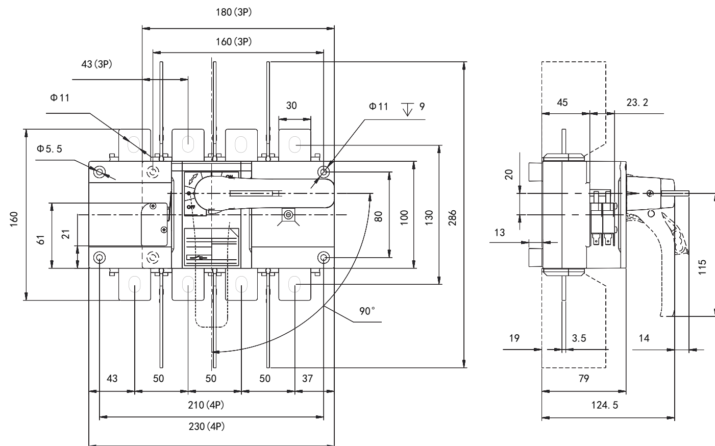
ГАБАРИТНЫЕ РАЗМЕРЫ ВН-IS-AKSOL 400AF С ВЫНОСНОЙ РУКОЯТКОЙ И КВВ
